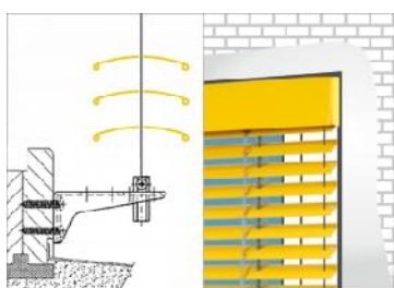
Vodící lanko (odsazení 50- 70 mm)
